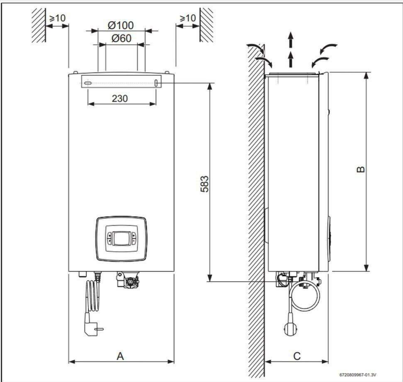
Мал. 1 Розміри (в мм)
