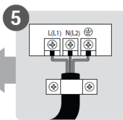
5 Підключіть дроти
